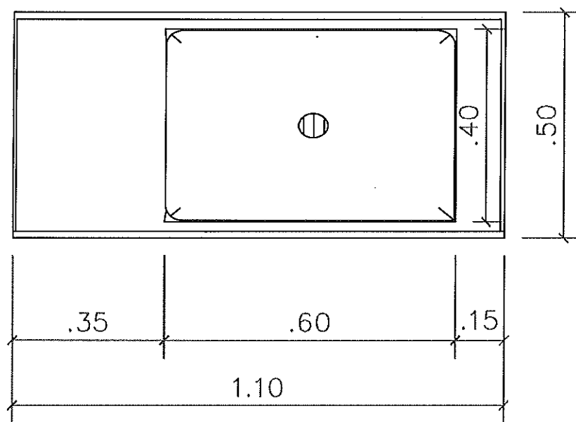
VISTA SUPERIOR
